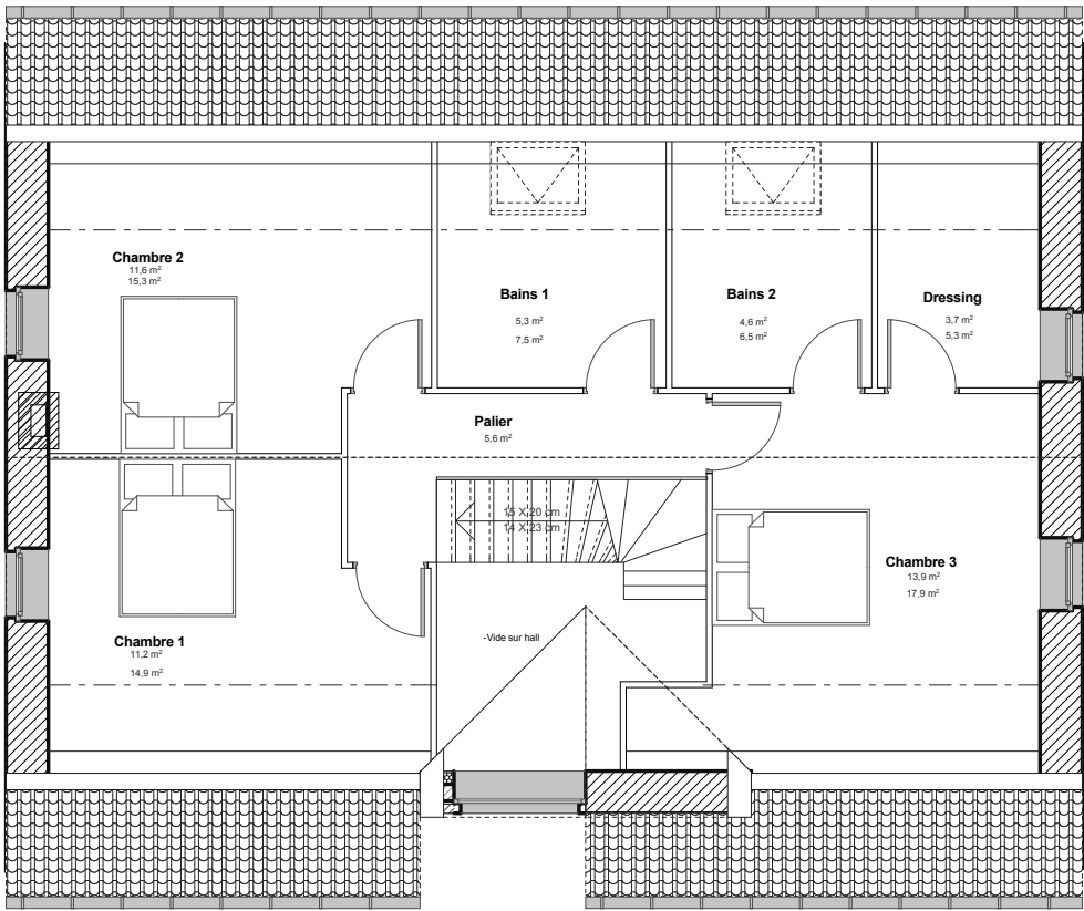
plan étage
