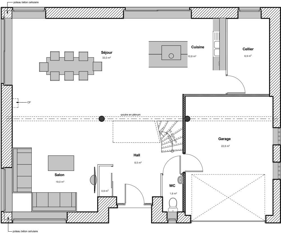
plan RDC
